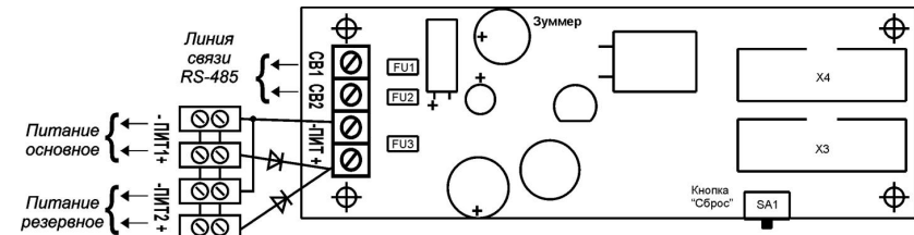
Рисунок 1 – Монтажная схема «Вертикаль-МИ»
