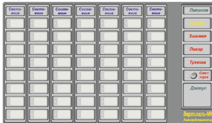
Рисунок 4 – Лицевая панель типового «Вертикаль-МИ» для систем адресной пожарной сигнализации
